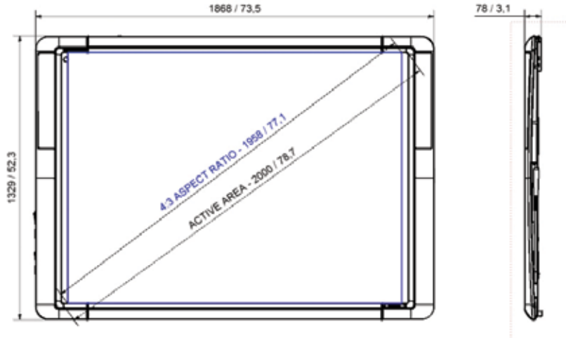
ActivBoard 378 Pro
